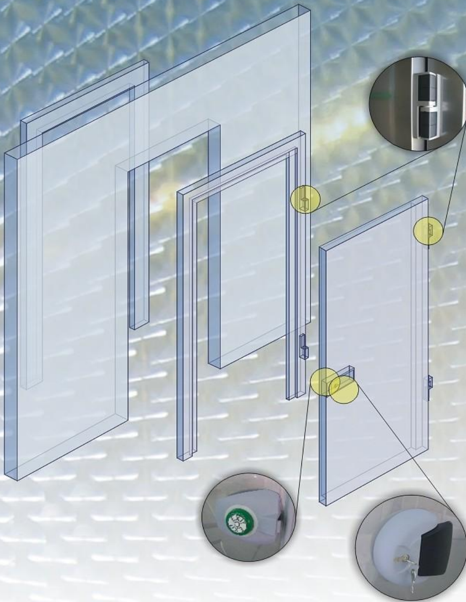
Hengslet dør med tosidig ramme.
